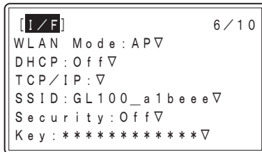
[I/F Setting]
