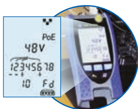
Service detectie
