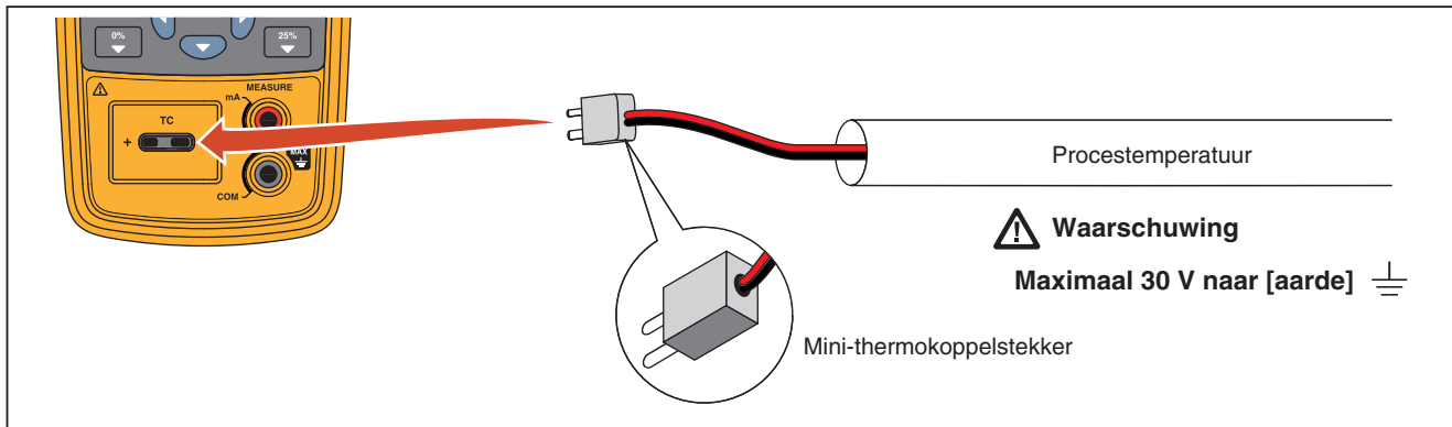
Afbeelding 6. Temperatuur meten met een thermokoppel
