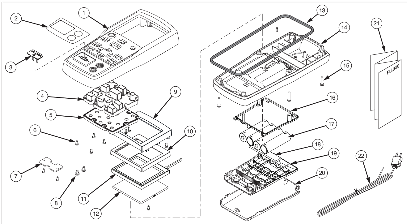
Abbeelding 9. Vervangingsonderdelen
