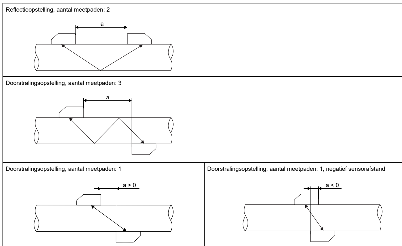
a - sensorafstand
